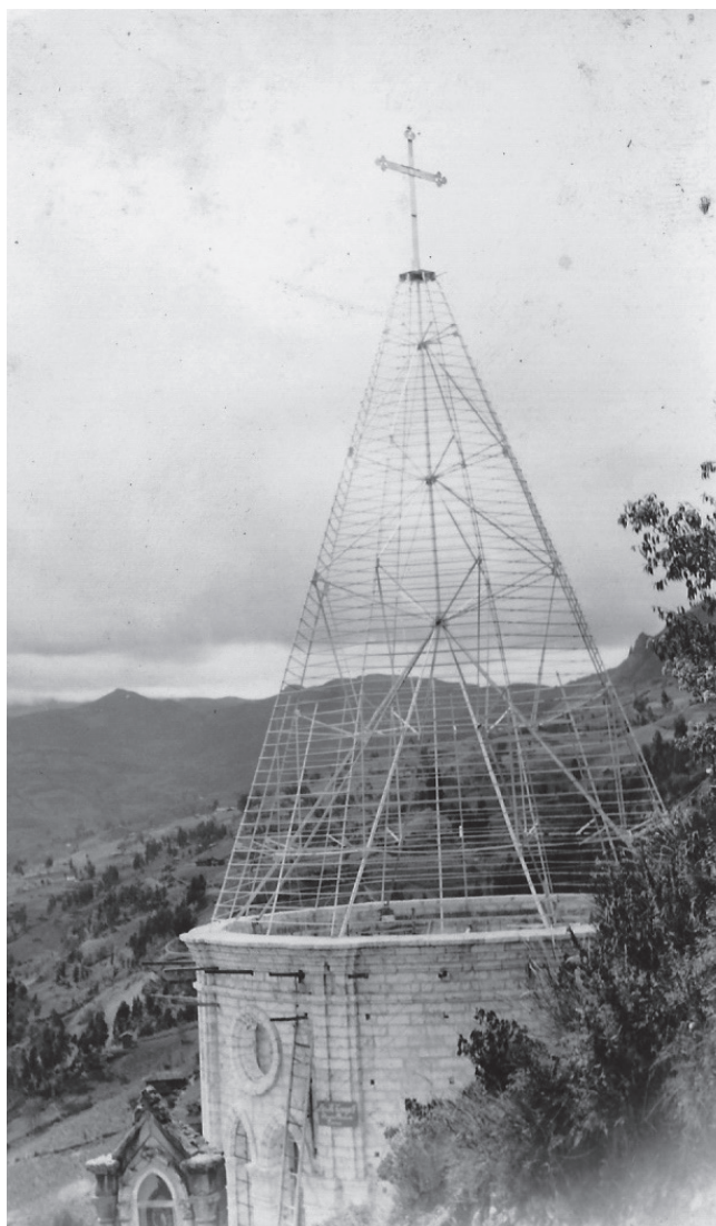
La estructura metálica de la primera cúpula del Santuario del Rocío fue diseñada por el ingeniero cuencano Rómulo Márquez. Foto: Derechos reservados del autor. 1960-1970.
