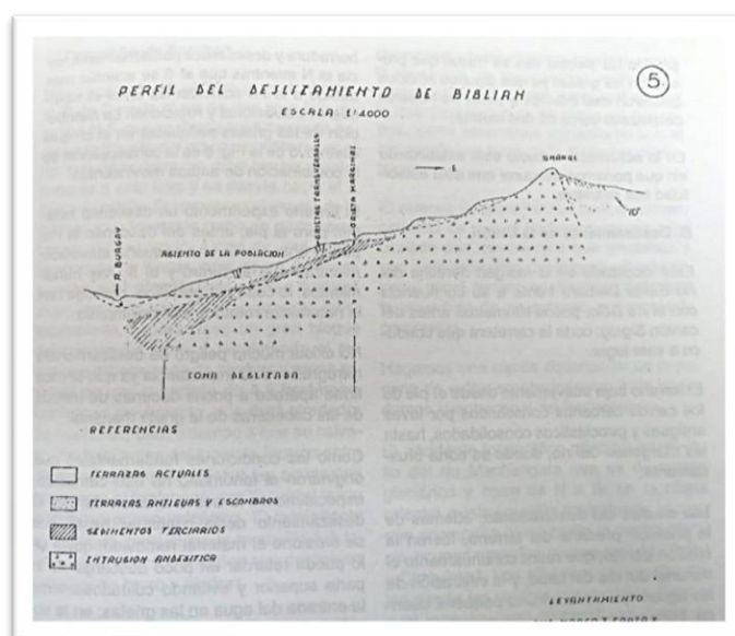
Plano del deslizamiento de las tierras en Biblián, año 1951. Autor: Ing. Marco Tulio Erazo.
